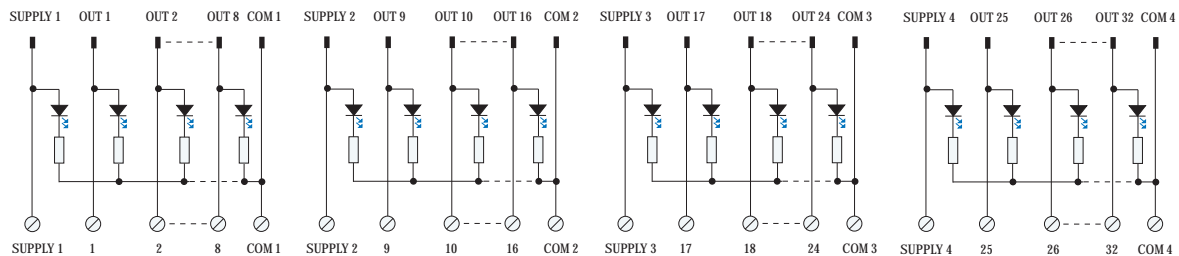
SCHEMA A BLOCCHI MODULI 32 USCITE - 32 OUTPUT MODULES BLOCK DIAGRAMS
